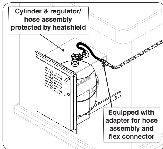
Fig. 10-3 Optional Fire Magic door w/tank tray
